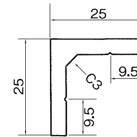
棚受け(AH-574)
